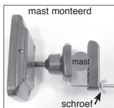
mast monteerd
