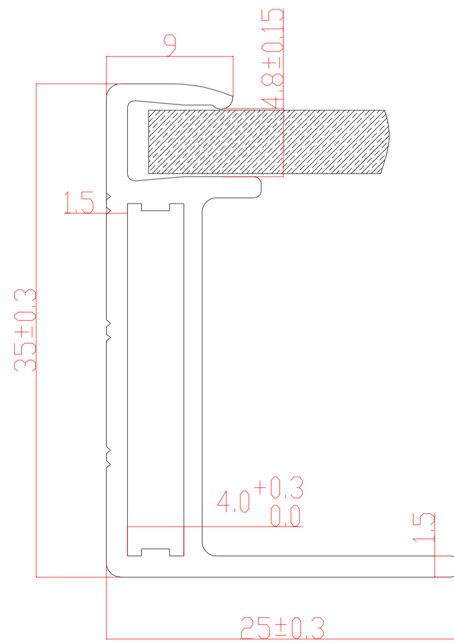
Schnitt A-A
